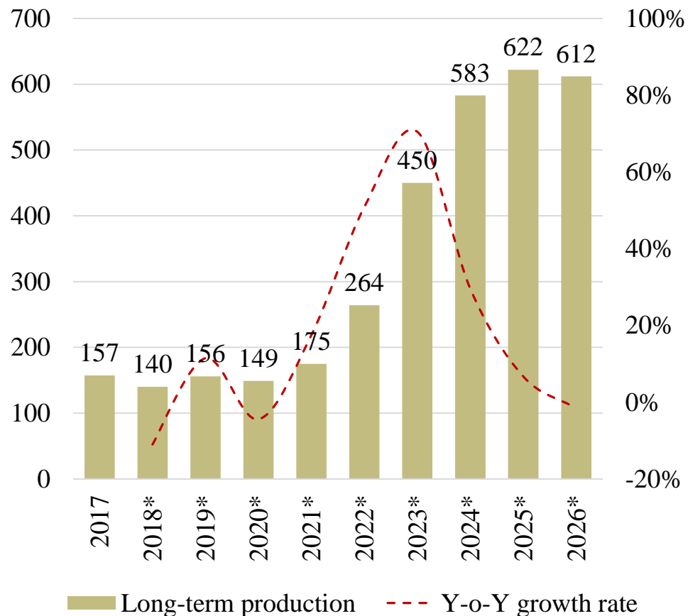
Оюу Толгойн зэсийн үйлдвэрлэлийн төлөвлөгөө
